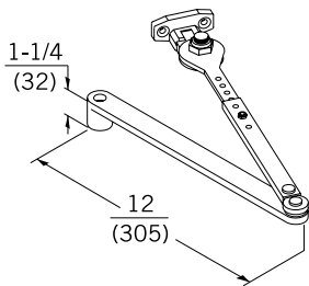
Opcional Brazo con retención de apertura FHP
